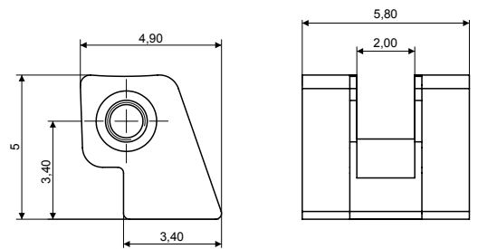
STEP HINGE
